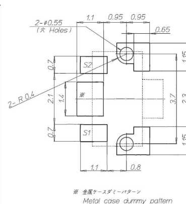
推奨はんだ付けパターン Recommendable soldering pattern
